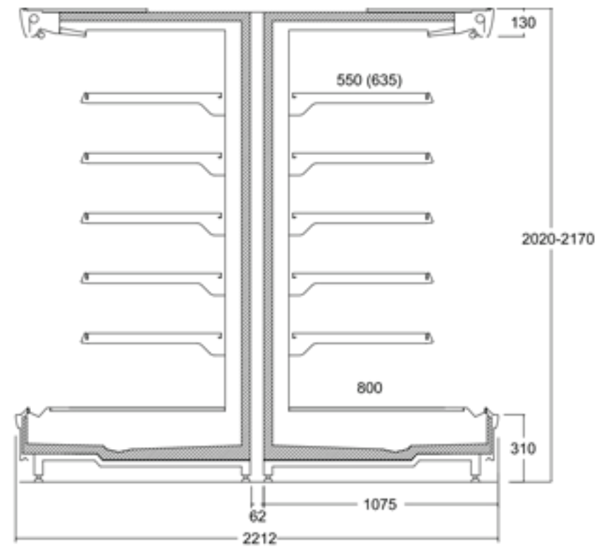
MERGA 107 GONDOL
