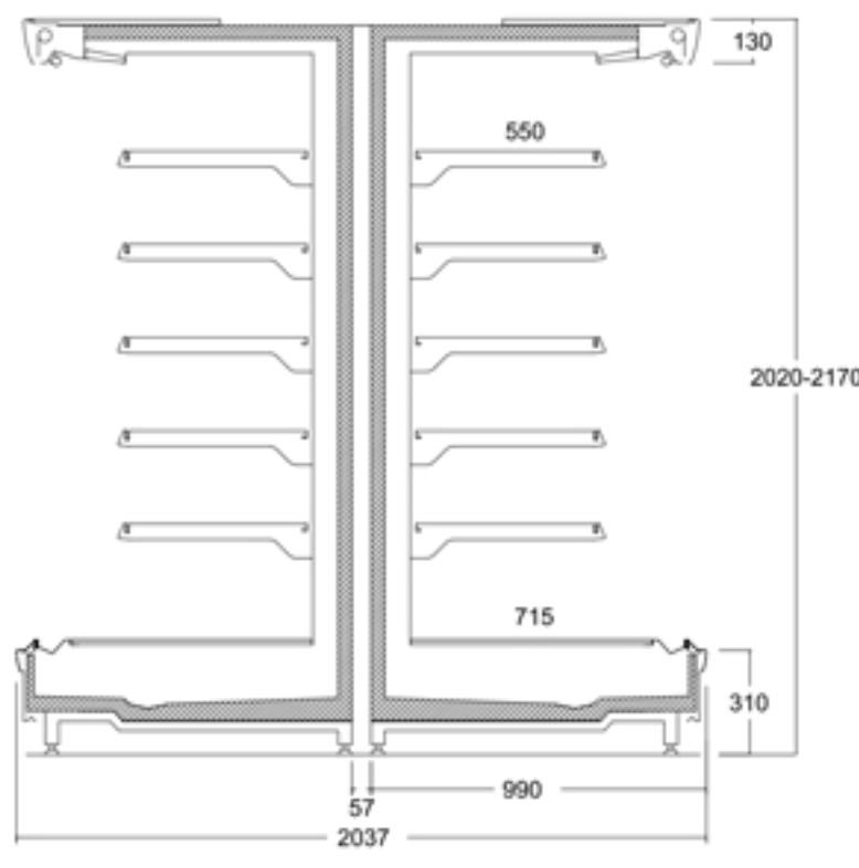
MERGA 99 GONDOL
